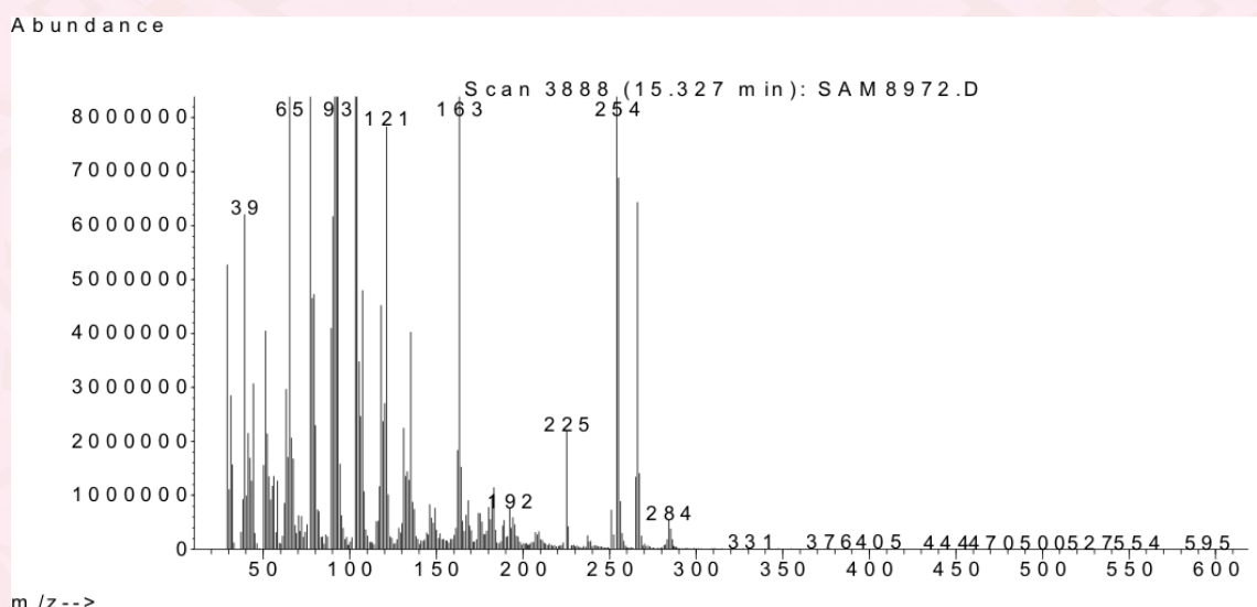
3-rasm. Tropikamidning mass-spektri
