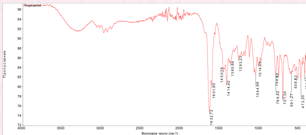
1-rasm. Tropikamidning IQ-spektri.
