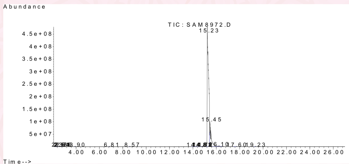
2-rasm. Tropikamidning xromatogrammasi
