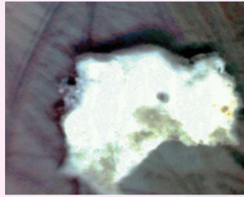
Картина отражения микрочастиц ЛКП в поле зрения интегрированного ИК-микроскопа Thermo Scientific Nicolet iN10 с встроенным микроскопом (размер частиц – до 100 мкм)
