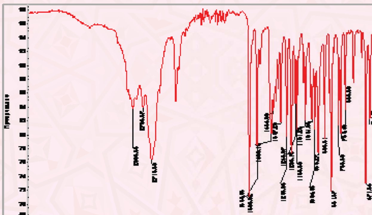
Рис. 3. ИК-спектр смыва из исследуемого пакетика
