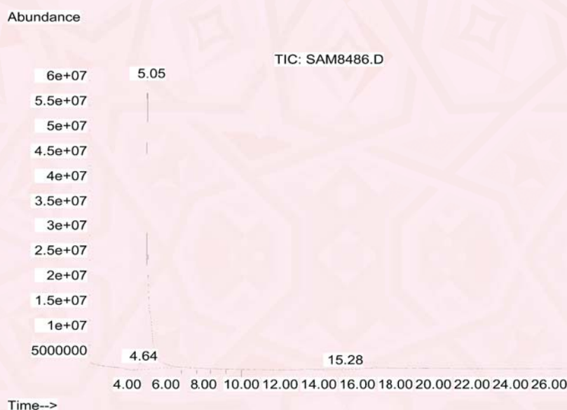
Рис. 1. Хроматограмма смыва из исследуемого пакетика
