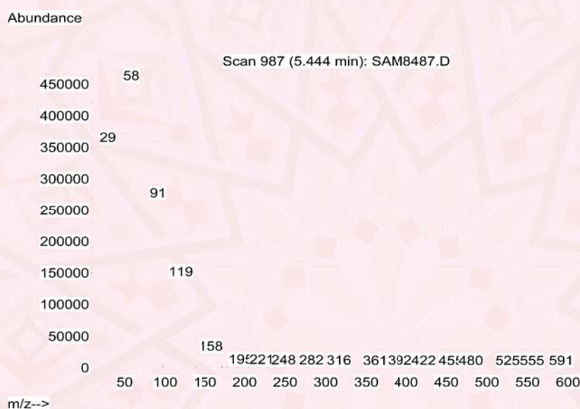
Рис. 2. Масс-спектр смыва из исследуемого пакетика
