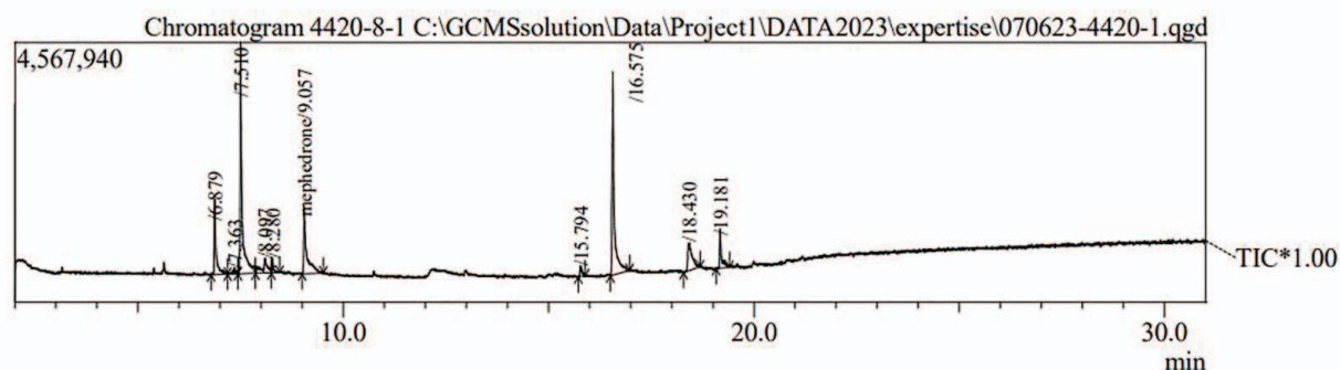
Рис. 4. Хроматограмма смеси мефедрона с тропикамидом и побочными продуктами синтеза.
