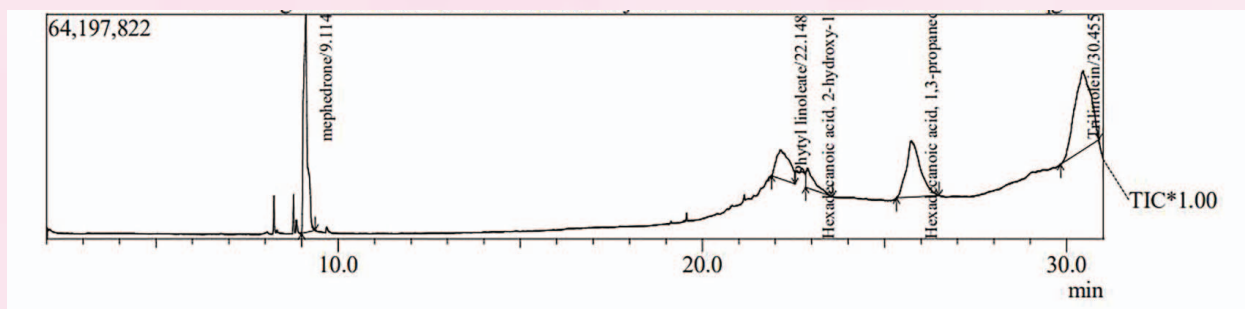
Рис. 6. Хроматограмма смеси мефедрона с наполнителем (крахмал) с побочными продуктами синтеза и сырьевыми компонентами
