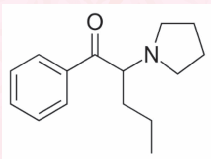
Рис. 1. Химическая структурная формула \alpha -PVP.
