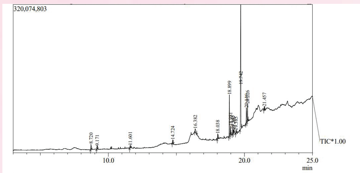
Рис. 5. Хроматограмма продуктов термического распада курительной смеси табака с примесями ТКК и \alpha -PVP
